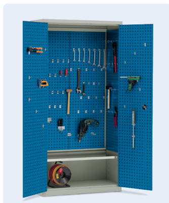
Varenr. 131V0007 MS-1 m. 1 galv. hyld og værktøjstavler på bagvæg, sider og låger Udv. mål i mm.: H:2000 B:1000 D:445 Lysningsmål i mm.: H:1870 B:920 D:425
