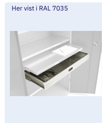
Varenr. 131T0002-7016 Udtræksskuffe m/teleskopudtræk for MS-1 og MS-0.5
