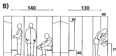
Anbefalet friplads i omklædningsrum med skabe, der har fast bänk. Ved lange rækker bør afstanden øges (cm).
