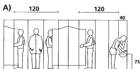
Arbejdstilsynets krav til friplads i omklædningsrum (cm).
