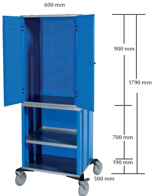
VERKTYGSVAGN TOOL TROLLEY Article no.800070
