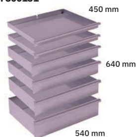
LÅDSATS 6 / DRAWER SET 6 Article no. 800131
