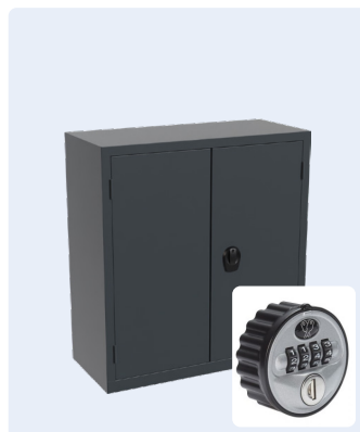
Varenr. 131V0011-218-7016-7016 MS-0.5 m. 2 galv. hylder og kodelås Eurolock 2800 Udv. mål i mm.: H:1075 B:1000 D:445 Lysningsmål i mm.: H:945 B:920 D:425
