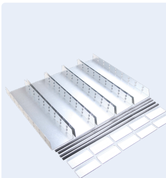
Varenr. 142T0080 Skuffeinddelingssæt i galv. stål til 131T0002 5 indsatsbakker, 10 stikvægge og 4 plastlister Indsatsbakke B: 167 mm. Stikvæg B:163 mm
