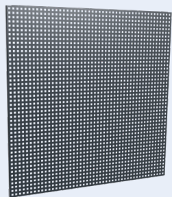
Varenr. 141F0025-7016 Værktøjstavle for MS-1 bagvæg 2 pr. skab. Med hul 10 x 10 mm Centerafstand 34 mm Udv. mål i mm.: H:1460 B:474 D:16
