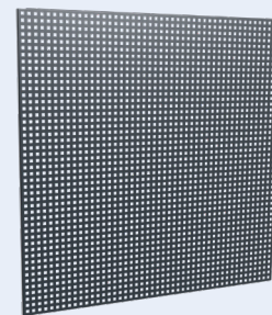
Varenr. 141F0019-7016 Værktøjstavle for MS-1 og MS-0.5 sider 2 pr. skab. Med hul 10 x 10 mm Centerafstand 34 mm Udv. mål i mm.: H:920 B:400 D:15
