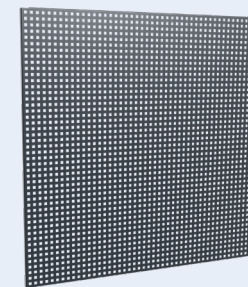
Varenr. 141F0013-7016 Værktøjstavle for MSG-3 midterskillevæg. Med hul 10 x 10 mm Centerafstand 34 mm Udv. mål i mm.: H:1460 B:400 D:14
