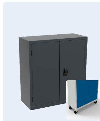
Varenr. 131V0011-S-7016-7016 MS-0.5 m. 2 galv. hylder og 80 mm. hjul Udv. mål i mm.: H:1180 B:1000 D:445 Lysningsmål i mm.: H:945 B:920 D:425
