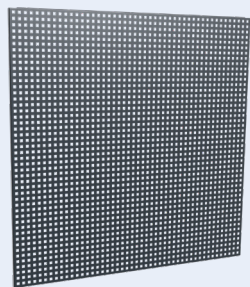
Varenr. 141F0011-7016 Værktøjstavle for MS-1 og MSG-3 højre side. Med hul 10 x 10 mm Centerafstand 34 mm Udv. mål i mm.: H:1460 B:400 D:17
