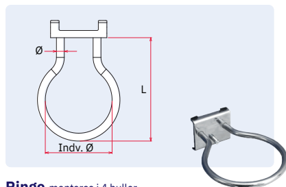
Ringe monteres i 4 huller
