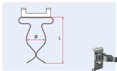
Fjederklemmer, standard monteres i 4 huller
