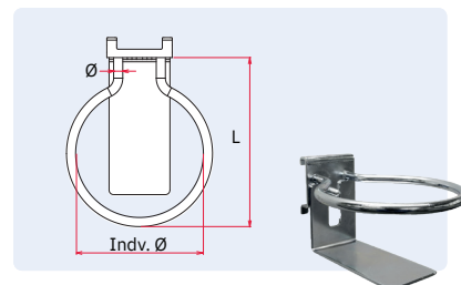
Smørekandeholder monteres i 4 huller
