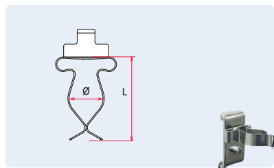
Fjederklemmer, standard
