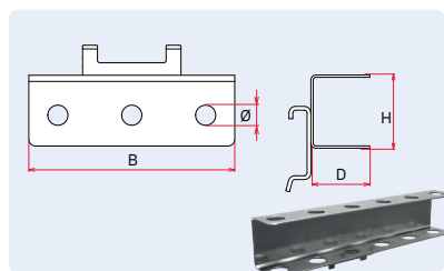
Skrutrækkerholder monteres i 4 huller
